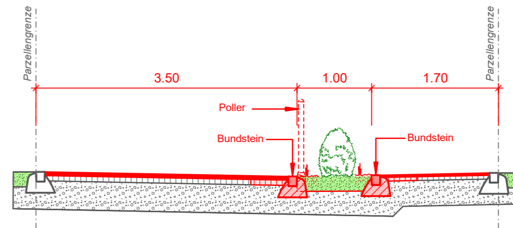
Einengung 1:50
