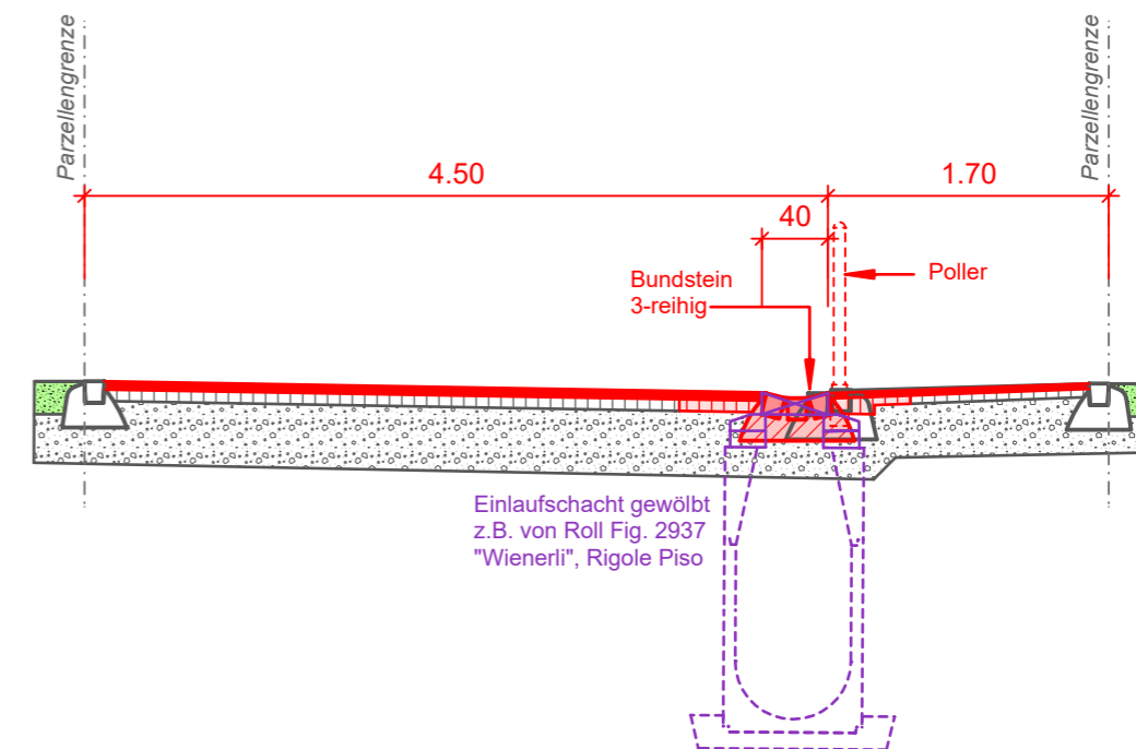
Strasse 1:50
